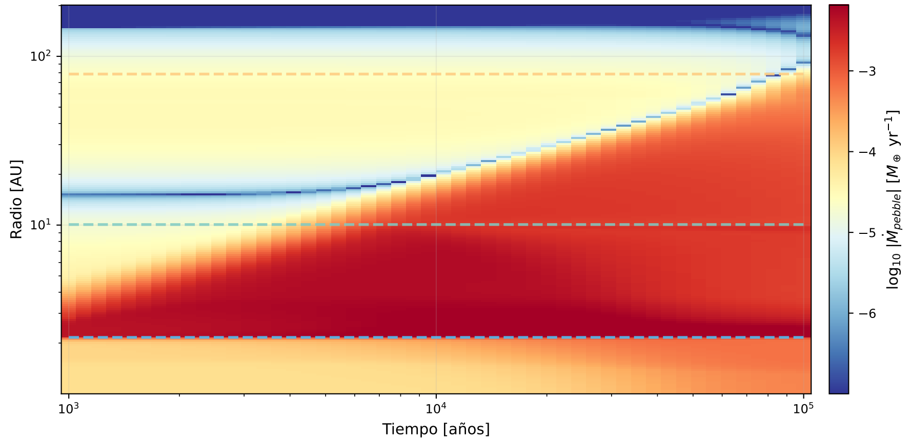
Flujo másico de Pebbles \dot{M}_{pebble}(r, t)
